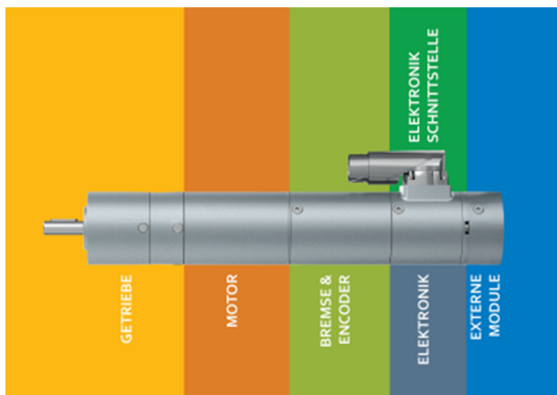
Bild 1: Die bisherige Palette des modularen Antriebssystems von ebm-papst mit 42 mm Durchmesser wird nun ergänzt um Motoren mit 63 mm Durchmesser und erstmalig auf der Motek vorgestellt.
